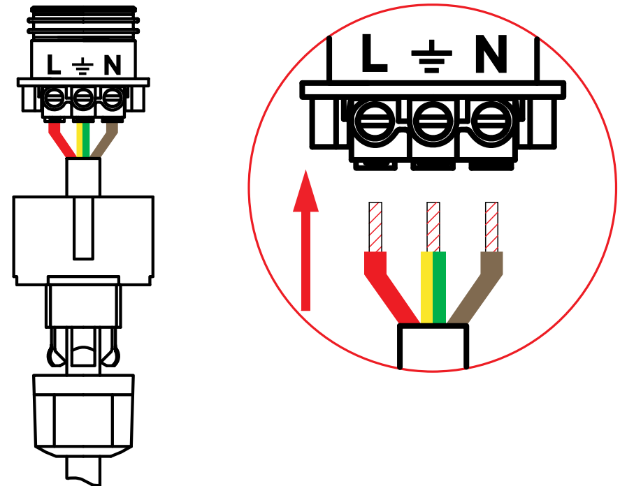
Рис.7 Схема подключения насоса.
